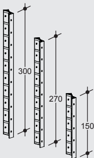
RASTO Gelenkecke 15/300* RASTO hinged corner 15/300*
