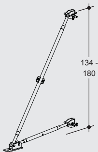
RASTO Justierstrebe RASTO adjusting strut
