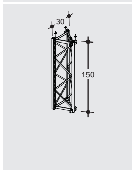
Dreieck Gittermast 1,5 m Lattice tower
