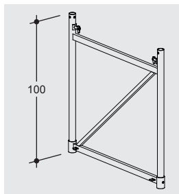
ID Normalrahmen 100 ID frame 100
