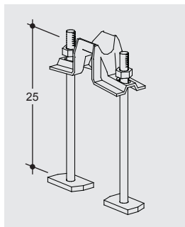
R 24 Drehgurtkupplung 250 Swivel clamp 250 R 24
