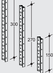
RASTO Gelenkecke 15/270 RASTO hinged corner 15/270
