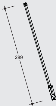
KG Stützstrebe KG bearer bar
