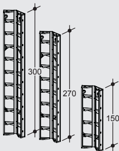
RASTO Gelenkecke 30/300* RASTO hinged corner 30/300*
