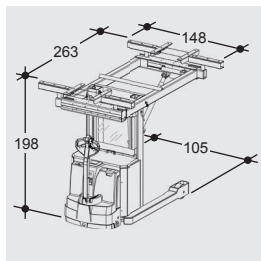
TOPMAX Tischhubwagen TOPMAX table jack lift
