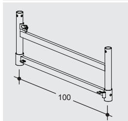
ID Ausgleichsrahmen 33 ID adjustment frame 33
