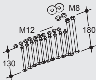
Schraubensatz CS 240 Screw set CS 240
