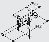
Widerlager f. Jochträger Adjustable abutment bracket
