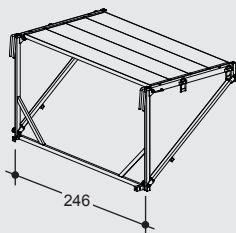
FALKO Konsolbühne 250 FALKO platform 250
