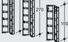
RASTO Gelenkecke 30/150* RASTO hinged corner 30/150*
