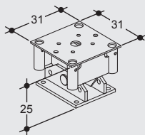
Gelenkfußstück Pin-jointed base plate
