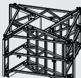
Säulenschalung 120/120 Column formwork 120/120
