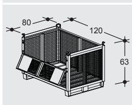
Euro Gitterbox Euro lattice box
