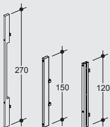
RASTO Eckausgleich 5/270 RASTO corner adjustment 5/270
