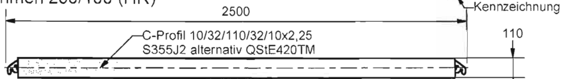
Horizontalrahmen 250/100 (HR)
