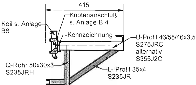
S-Konsolriegel
