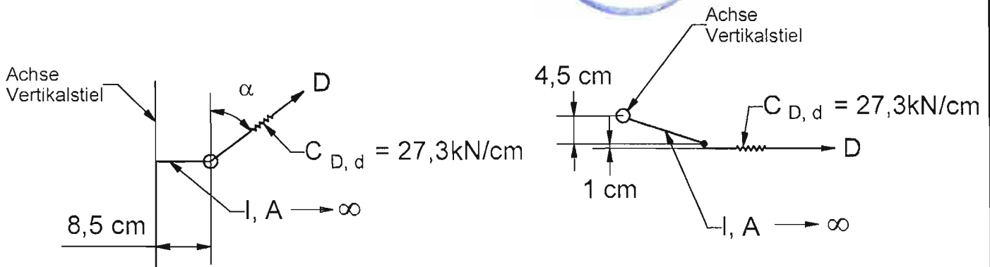
Bild 2: Statisches System Vertikaldiagonalanschluß
