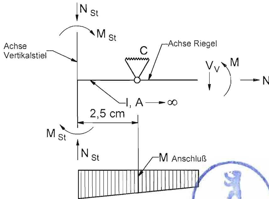
Bild 1: Statisches System Riegelanschluß
