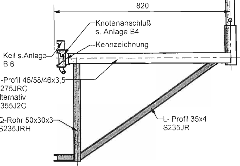
Konsole 82 A
