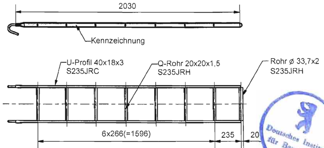
Leiter 200 hoch
