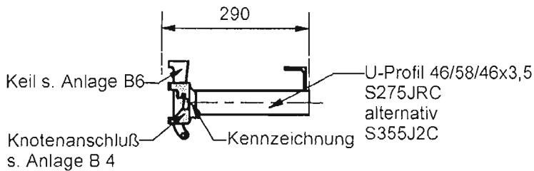
S-Riegel
