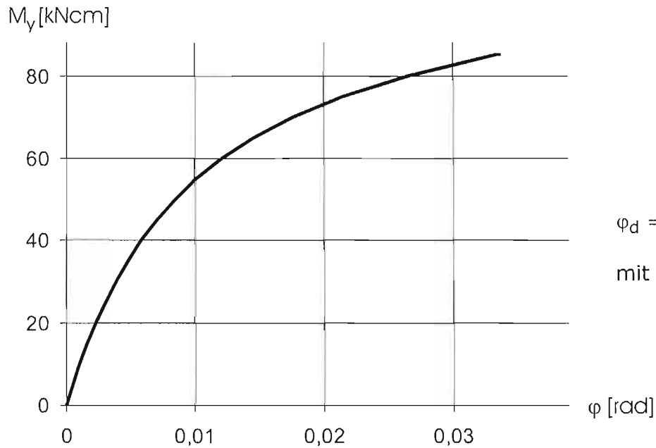
Bild 4: Drehfedersteifigkeit im Riegelanschluss
