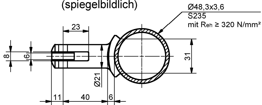
Gabelbolzen S235
