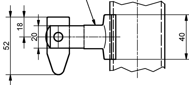
Gabelbolzen S235
