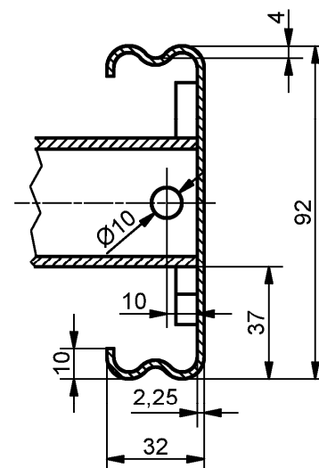
Schnitt Y-Y
