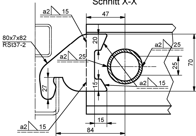
Schnitt X-X
