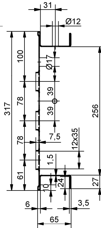
Ansicht A
