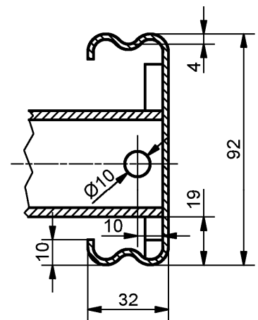
Schnitt Y-Y
