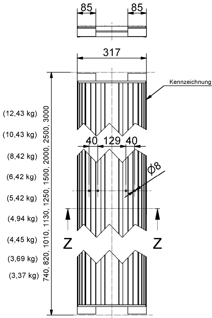
Schnitt Z-Z
