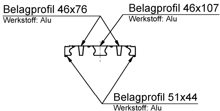
Schnitt Z-Z
